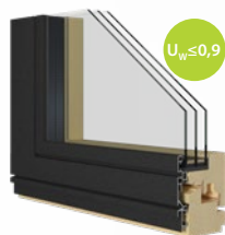
Premium PROFILO IN LEGNO + MASCHERA IN ALLUMINIO 68 mm + maschera
