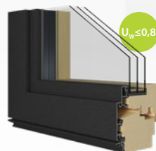
Premium PROFILO IN LEGNO + MASCHERA IN ALLUMINIO 92 mm + maschera
