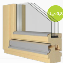
PROFILO IN LEGNO 94 mm
