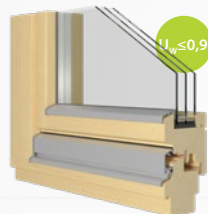
PROFILO IN LEGNO 68 / 84 mm
