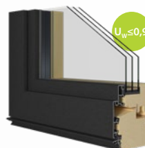
Premium PROFILO IN LEGNO + MASCHERA IN ALLUMINIO 94 / 78 mm + maschera
