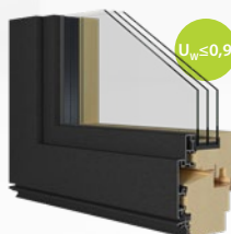
Premium PROFILO IN LEGNO + MASCHERA IN ALLUMINIO 78 mm + maschera
