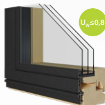
Premium PROFILO IN LEGNO + MASCHERA IN ALLUMINIO 92 mm + maschera
