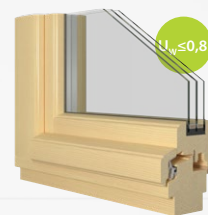
DRVENI PROFIL 68, 78, 92 mm
