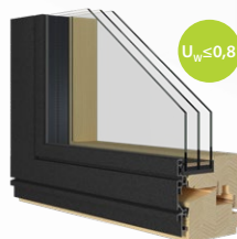
Premium DRVENI PROFIL + ALU MASKA 92 mm + alu maska
