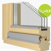
DRVENI PROFIL 94 mm
