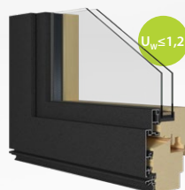
Premium DRVENI PROFIL + ALU MASKA 68 mm + alu maska
