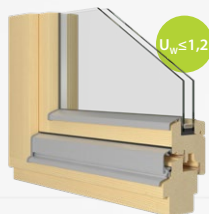
DRVENI PROFIL 68 mm
